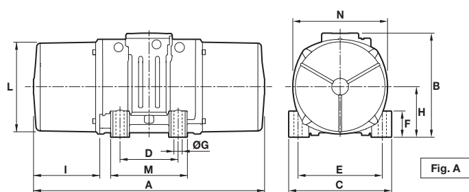
Dimensiones (mm)
