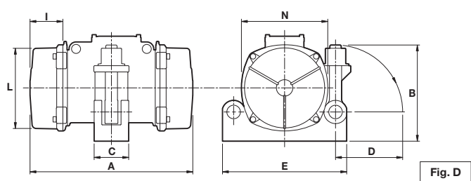
Dimensiones (mm)
