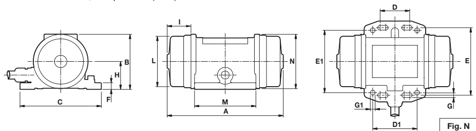
Dimensiones (mm)
