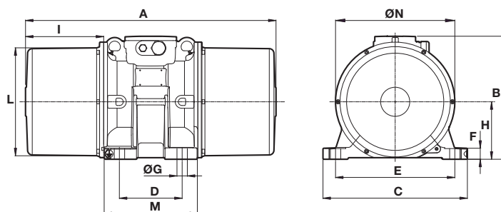
Dimensiones (mm)
