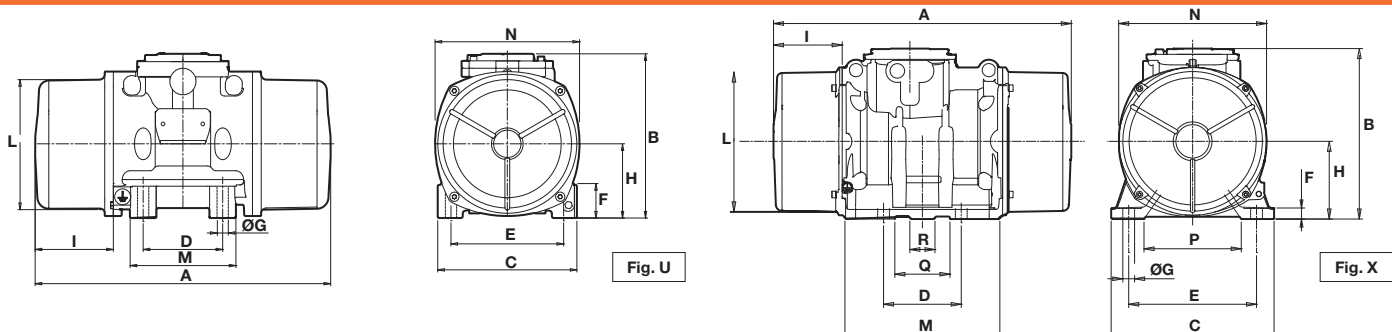
Dimensiones (mm)
