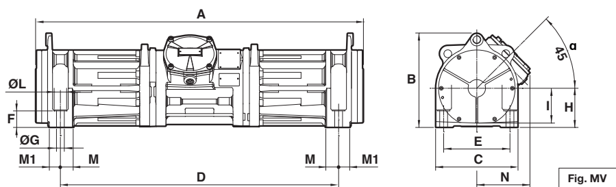
Dimensiones (mm)
